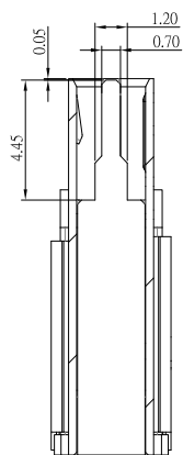
剖視圖
